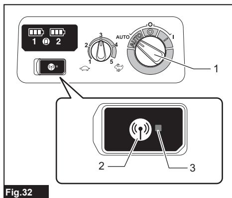
► 1. Interruptor de modo en espera 2. Botón de activación inalámbrica 3. Luz indicadora de activación inalámbrica
